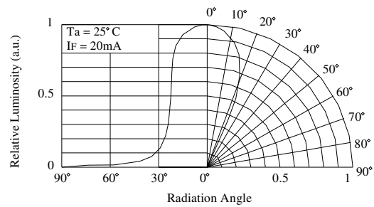
Directivity (Angle : 45^\circ )
