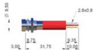
SOLDER LUG/FASTONS
